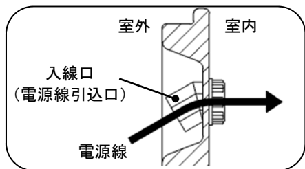
入線口詳細
