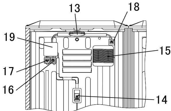
Fig. 1-3 室内左室配線周辺イラスト
