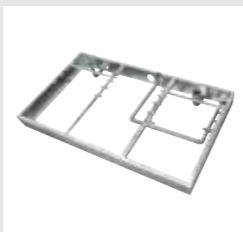
排水ユニット ※お客様にて現地取付となります。 ※水洗タイプのみ対応となります。 3室タイプ:W2850×D1630×H250 2室タイプ:W1910×D1630×H250
